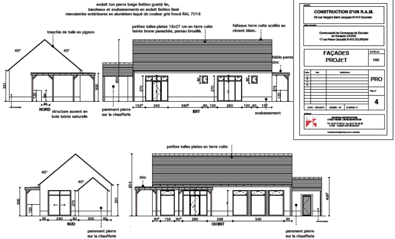
PLAN de façade du projet.
